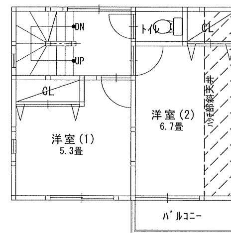
3 階 平 面 図 S = 1 : 1 0 0
